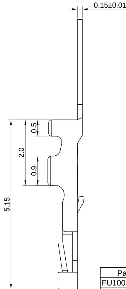
SEC: A-A
