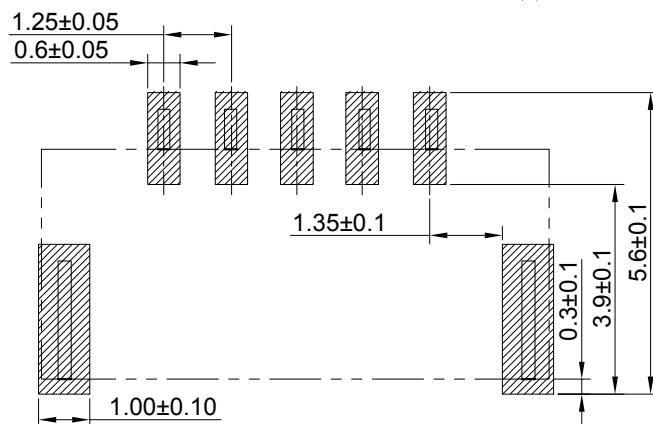
P.C.B LAYOUT
