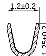
SEC:B-B
