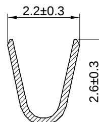
SEC A-A
