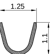
SEC A-A
