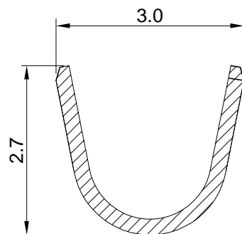
SEC A-A
